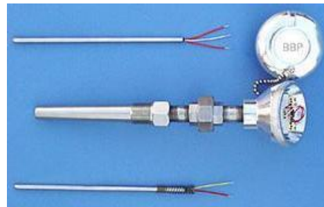
Thermocouple/Thermowell Assembly
